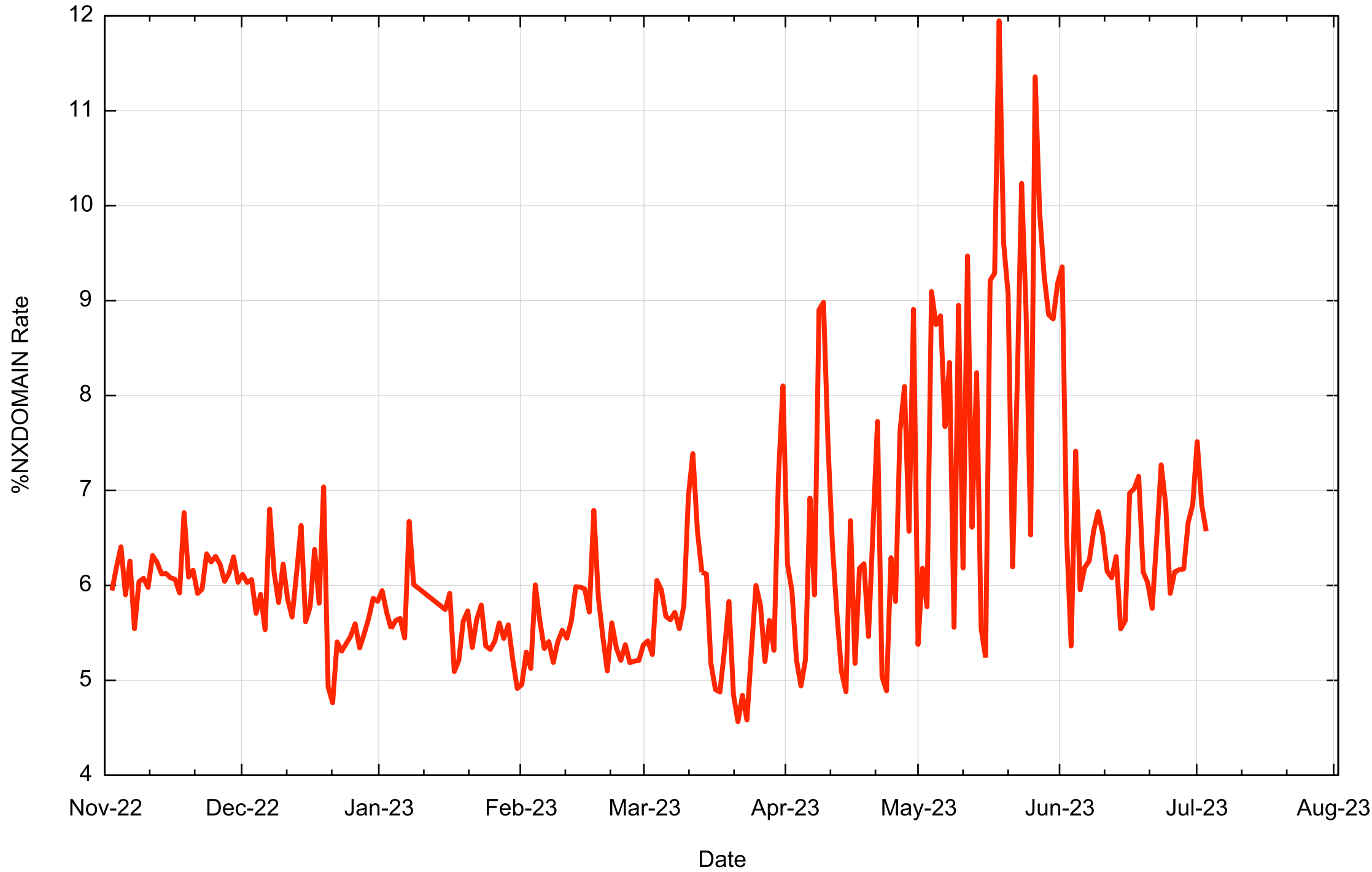
1.1.1.1 NXDOMAIN Ratio
