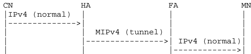
(d) MIPv4: CN-->MN, Foreign agent CoA
