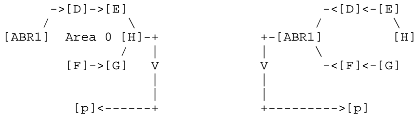
(d) MRT-Blue in Area 0 (e) MRT-Red in Area 0
