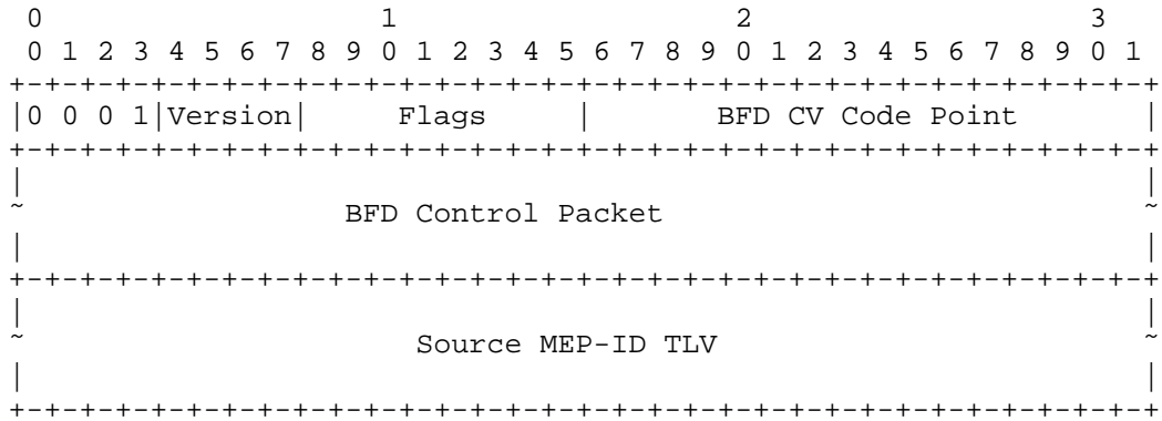
Figure 3: MPLS-TP CV Message
