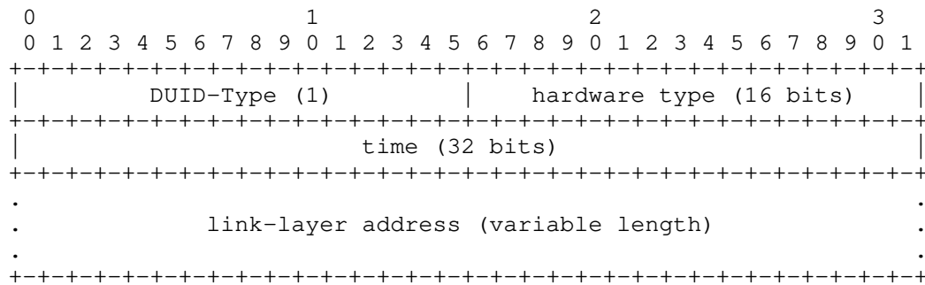
Figure 4: DUID-LLT Format
