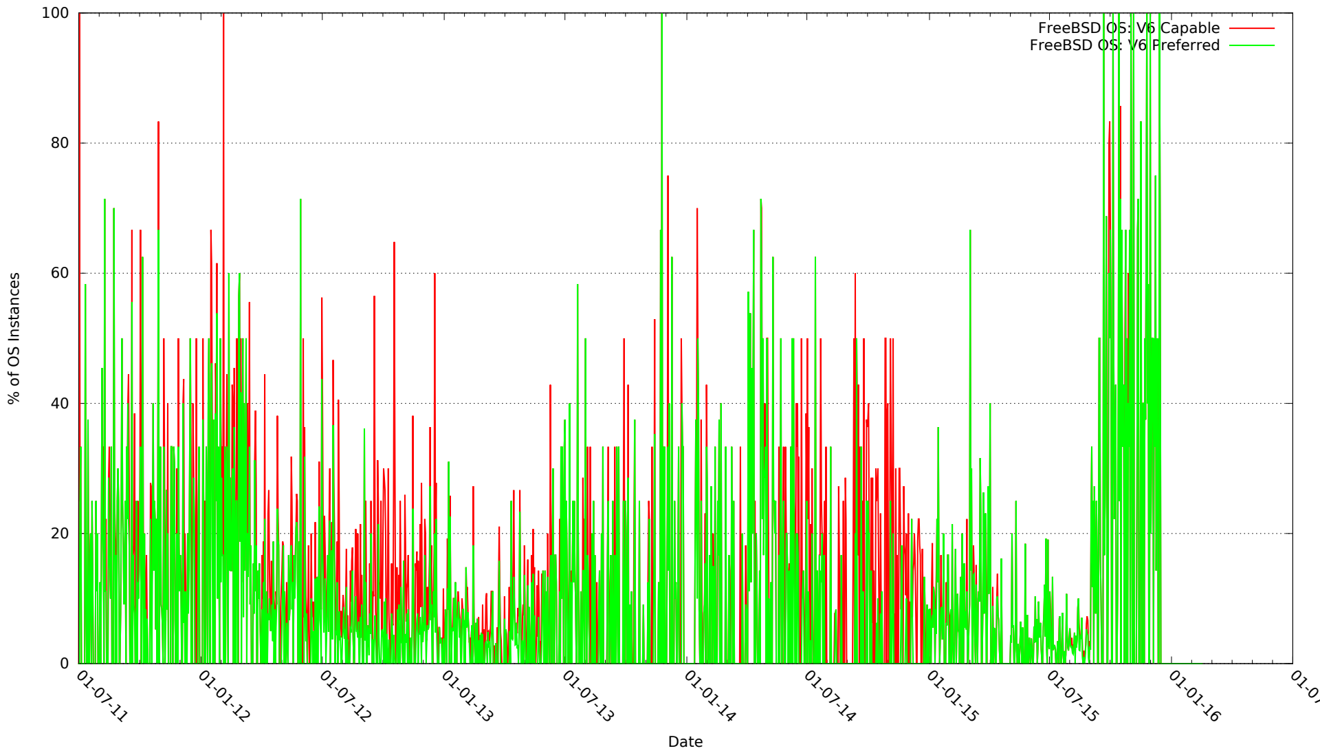
V6 FreeBSD OS Capability
